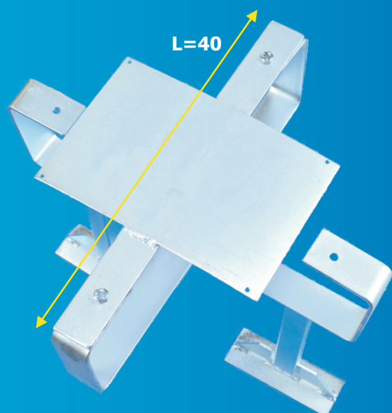
stelaż na kabel, słup EPV, L.40, ocynk
