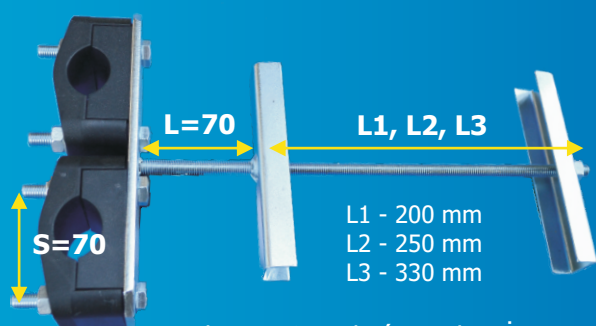
uchwyt KO podwójny, słup ŻN rozmiar 40, ocynk
