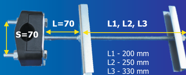
uchwyt KO pojedynczy, słup ŻN rozmiar 40, ocynk
