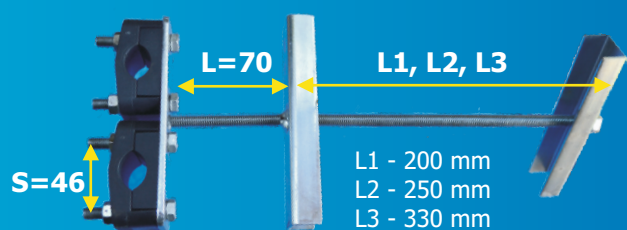
uchwyt KO podwójny, słup ŻN rozmiar 27, ocynk
